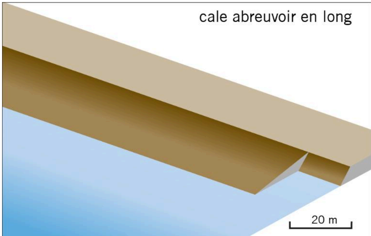
Schéma d'une cale à abreuvoir en long.
